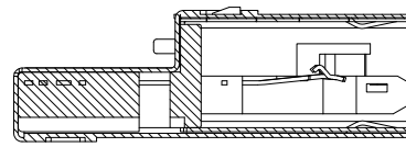
目检标准: 端子头部低于塑胶面 剖面 A-A
