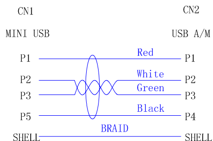
Wire Diagram:
