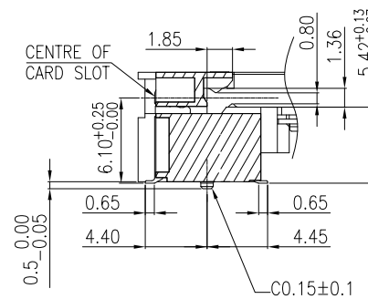
SECTION:A-A SCALE 2:1
