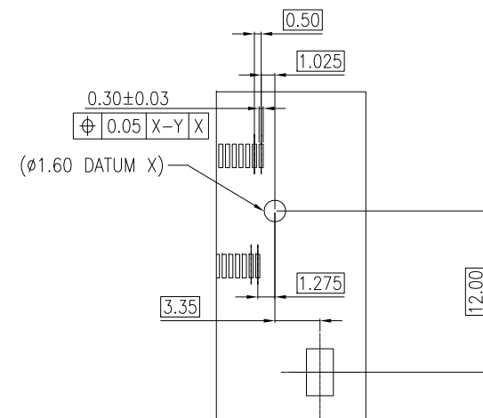
DETAIL:D SCALE 2:1
