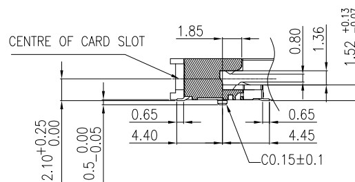
SECTION:A-A SCALE 2:1
