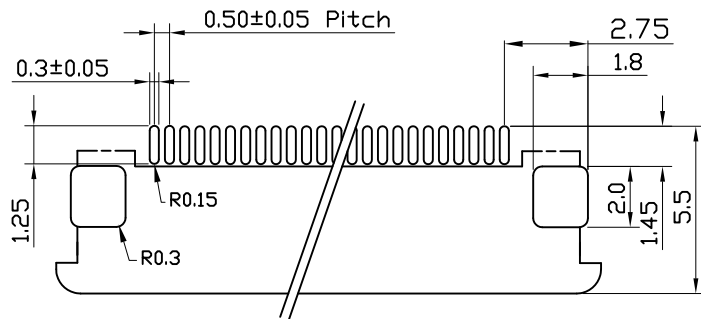
P.C.B Layout
