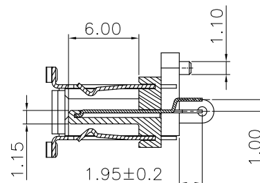
SECTION A-A 1:1
